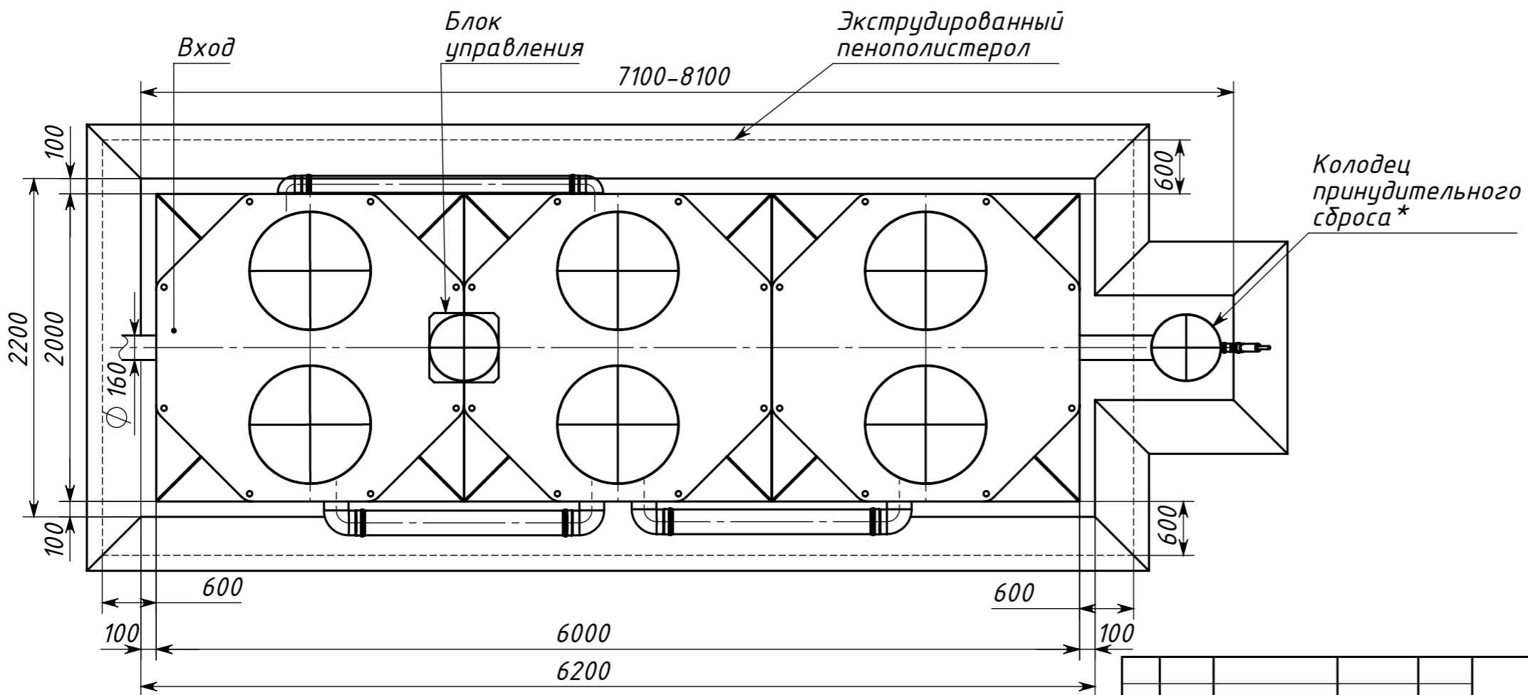
Вид сверху
